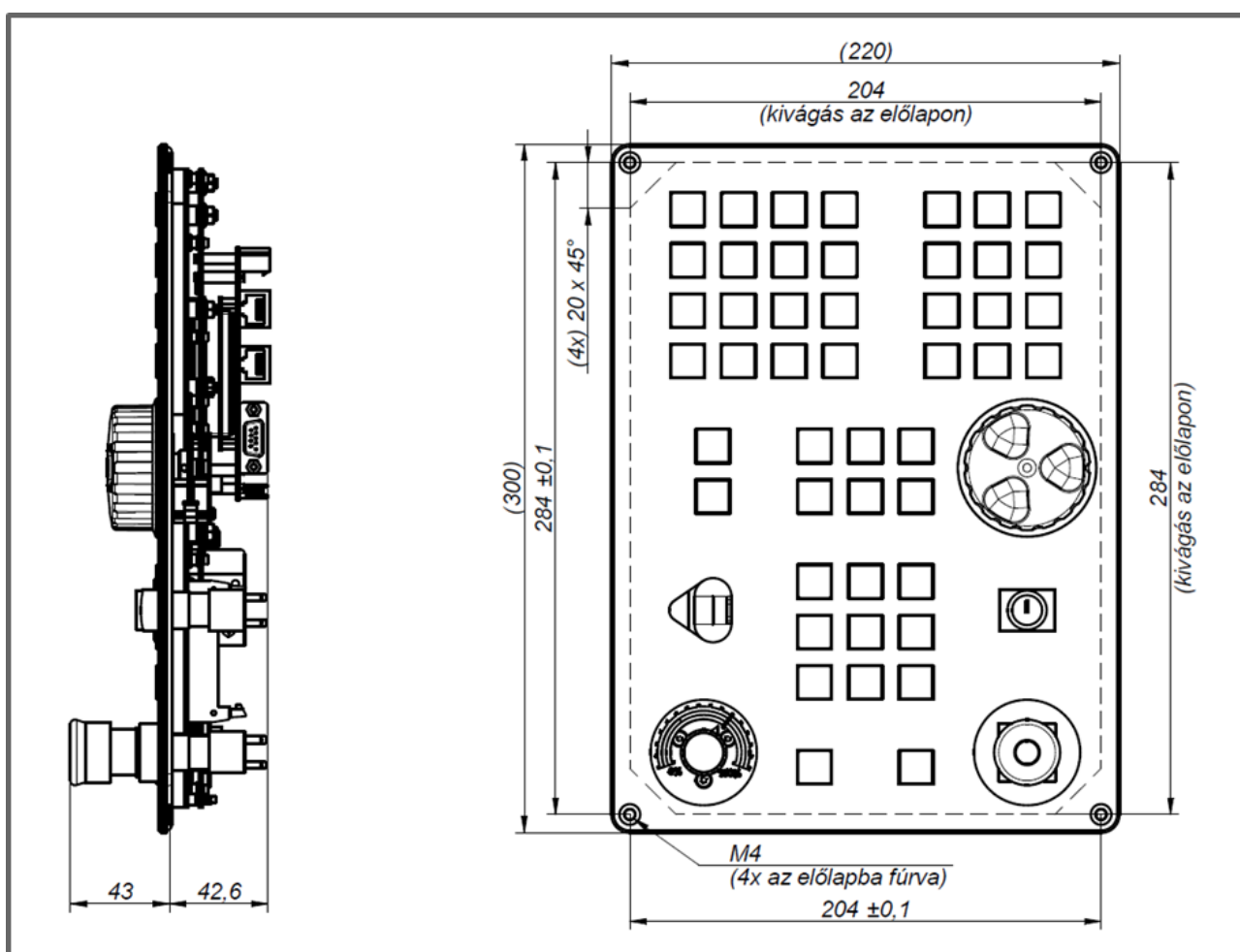
MK15CV PANEL KÖRVONALRAJZ
