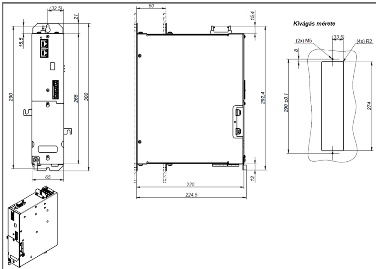
PDC-3-40-24 / PDC-3-40-24-R TÁPEGYSÉG KÖRVONALRAJZA
