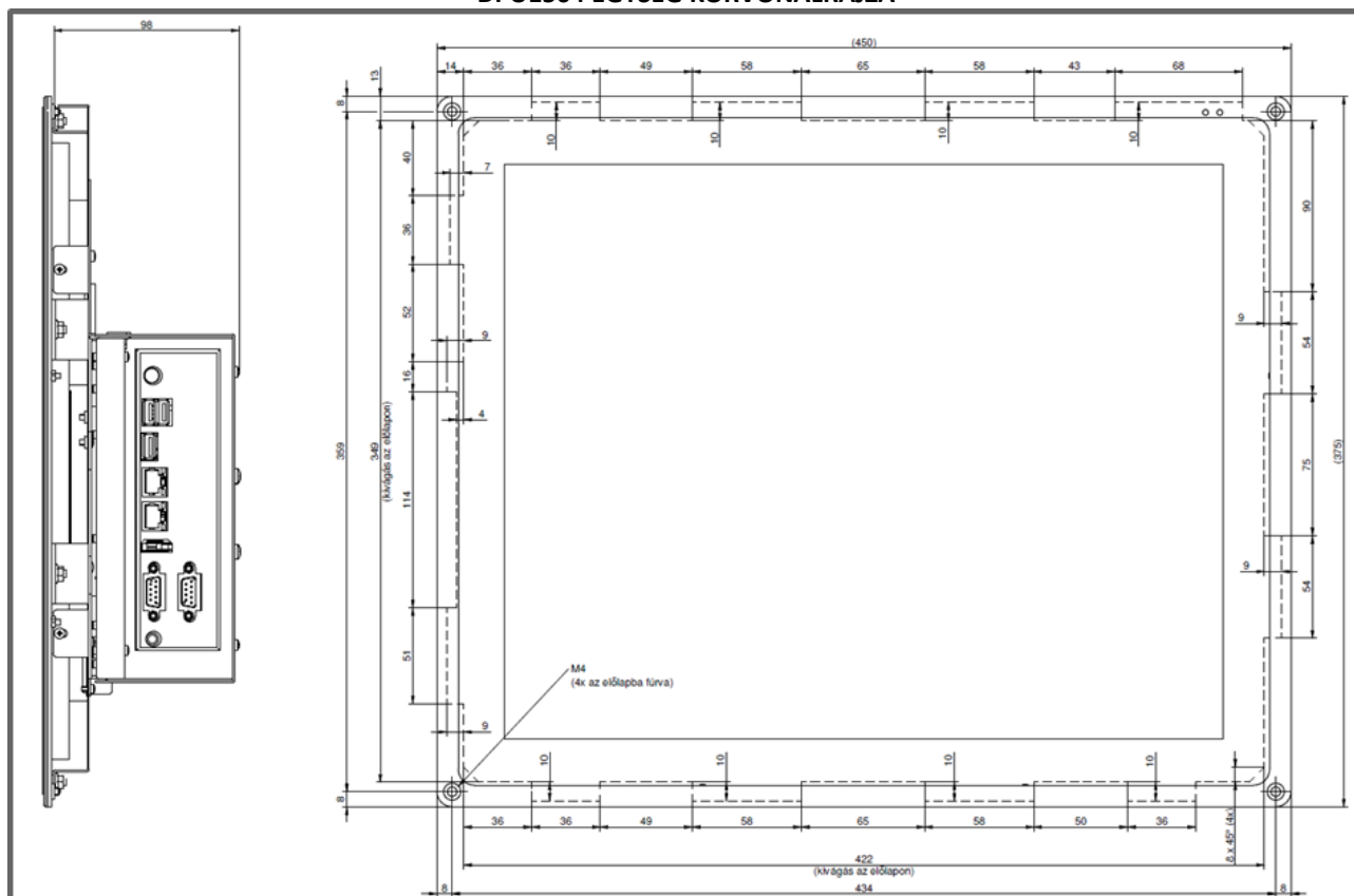
DPU1904 EGYSEG KÖRVONALRAJZA
