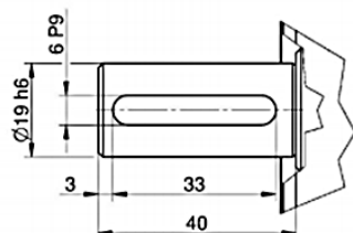
Hengeres, reteszhomyos tengelyvég
