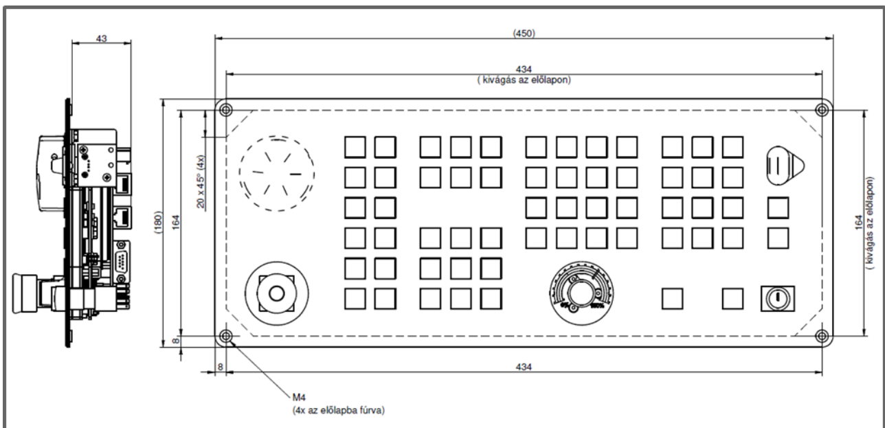
MK1904 PANEL KÖRVONALRAJZA
