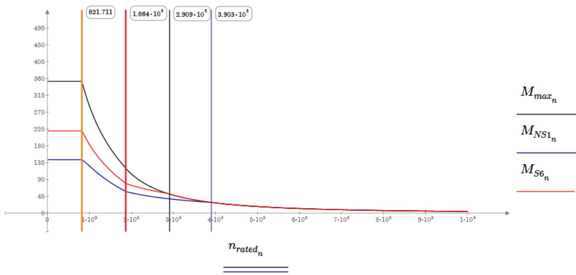
3. ábra AiS132LW08-15H motor nyomatéka Y kapcsolásban
