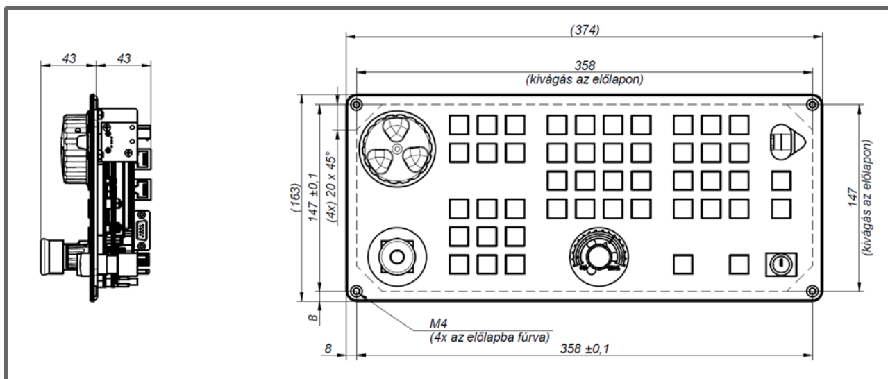
MK15C PANEL KÖRVONALRAJZ
