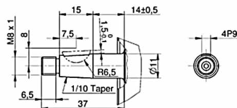
Kúpos tengelyvég
