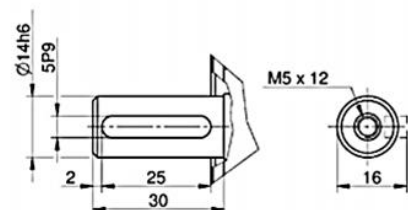
Hengeres, reteszhorvostengelyvég
