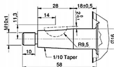
Kúpos tengelyvég
