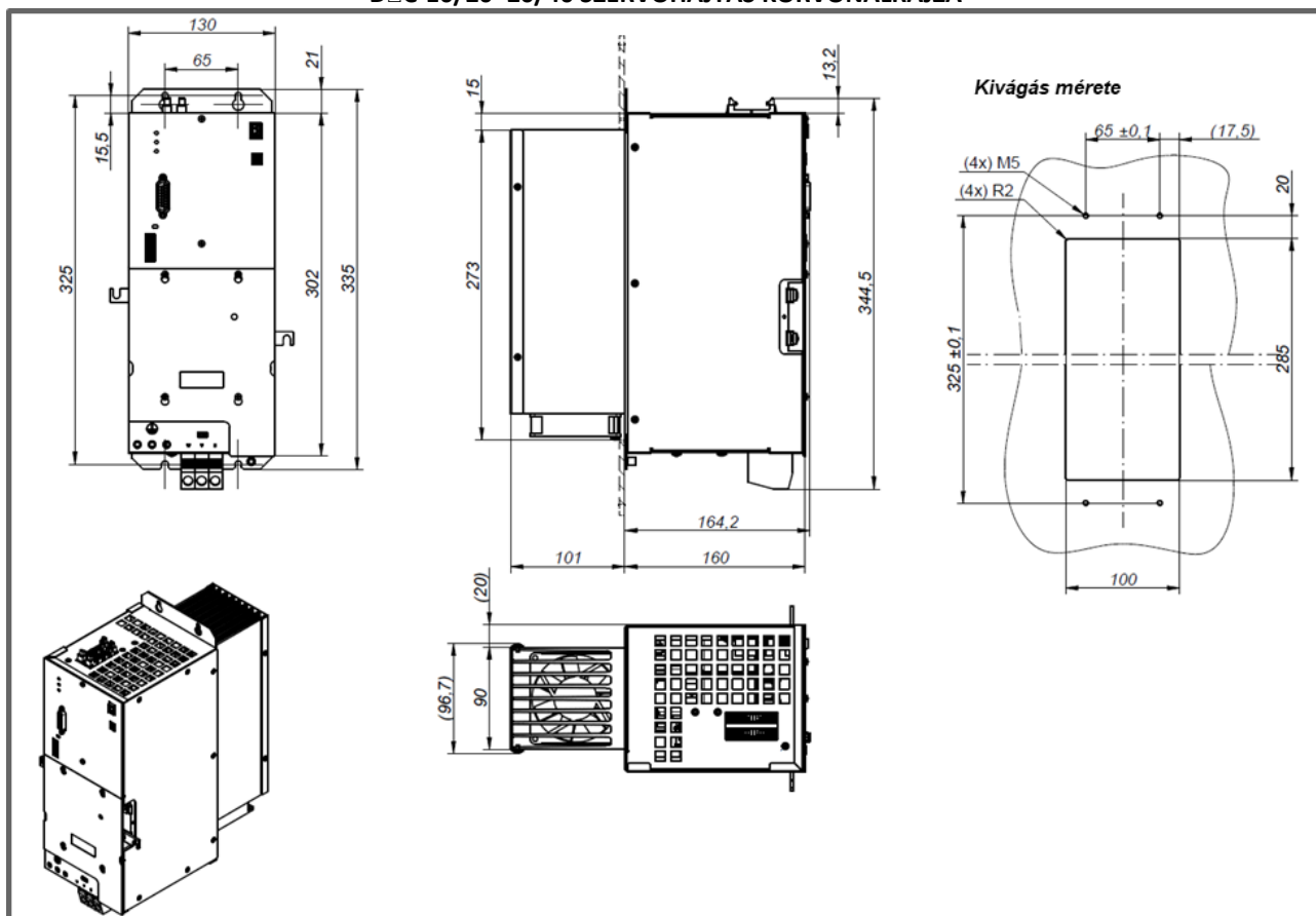
D□C-40/80~60/120 SZERVOHAJTÁS KÖRVONALRAJZA
