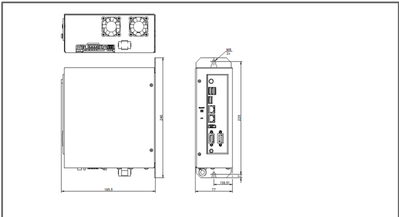
EHU04B EGYSÉG KÖRVONALRAJZA
