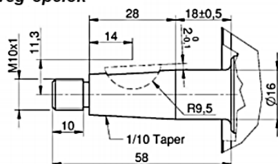
Kúpos tengelyvég
