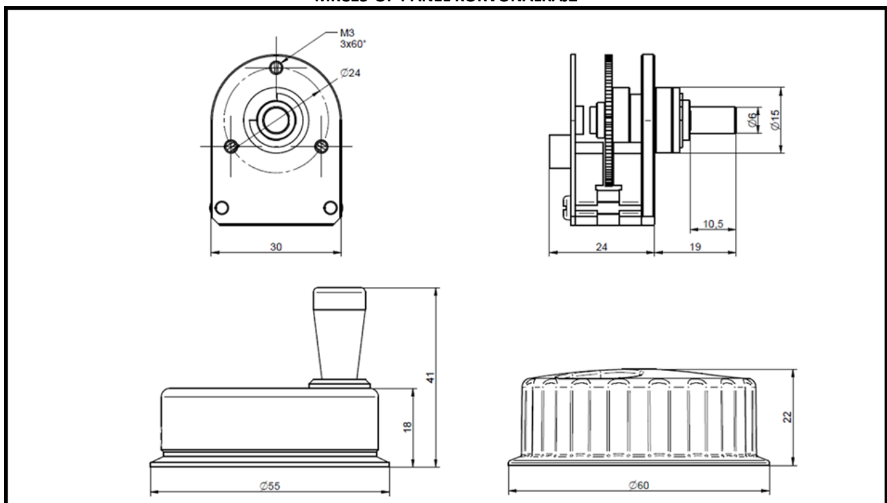
HWM KÉZIKERÉK KÖRVONALRAJZA
