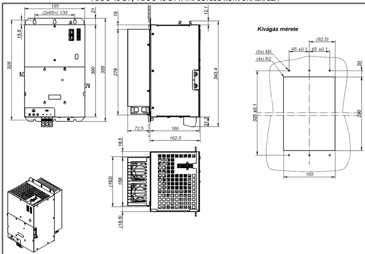
PRC-3-40-80-R TÁPEGYSÉG KÖRVONALRAJZA
