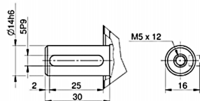
Hengeres, reteszhorvostengelyvég
