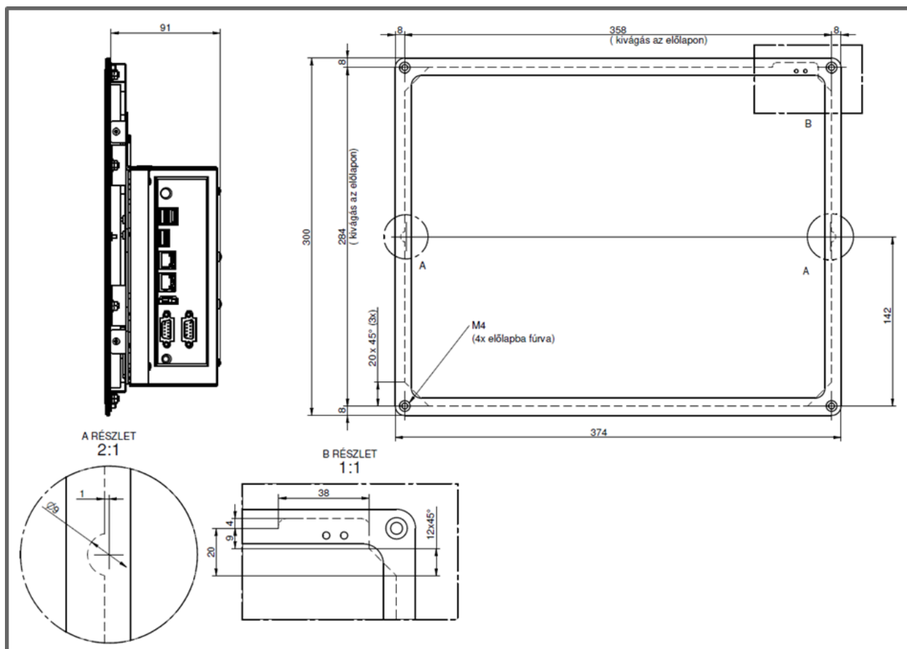
DPU1504 EGYSÉG KÖRVONALRAJZA
