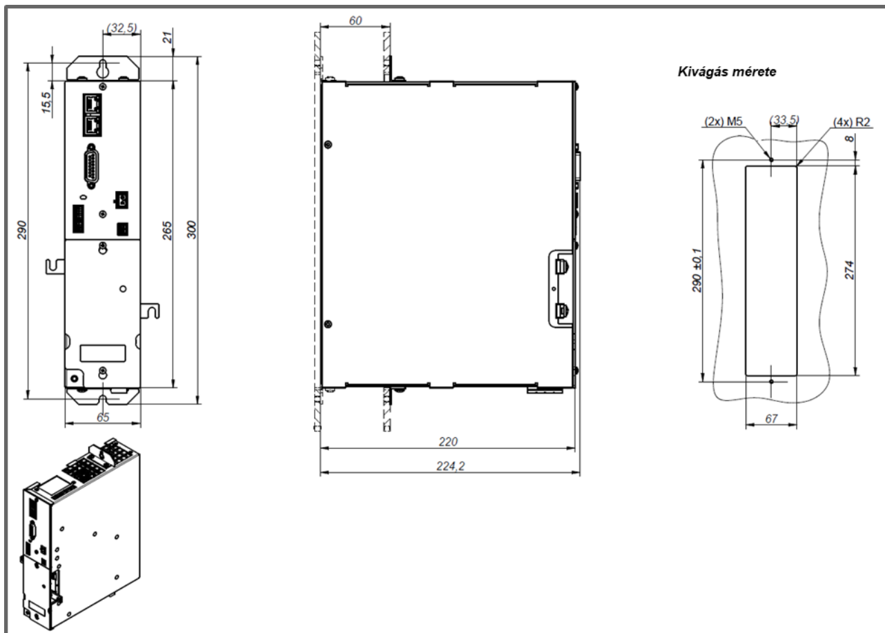
D□C-10/20~20/40 SZERVOHAJTÁS KÖRVONALRAJZA
