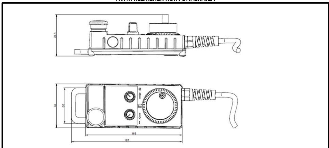
iHDW KIHELYEZETT KÉZIKERÉK KÖRVONALRAJZA
