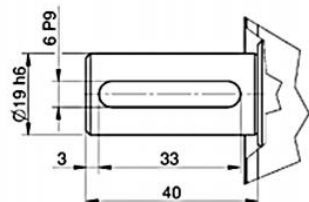
Hengeres, reteszhomyos tengelyvég
