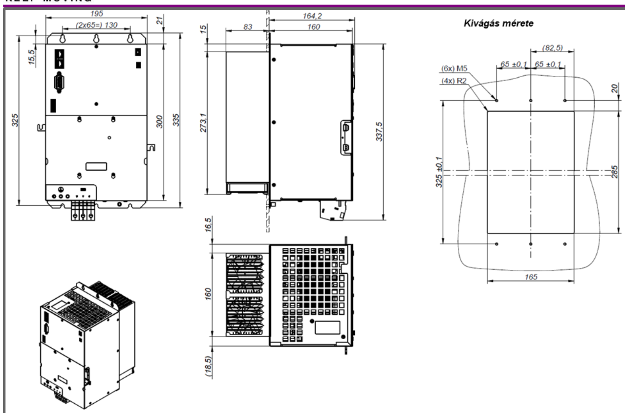
D□C-80/160 SZERVOHAJTÁS KÖRVONALRAJZA
