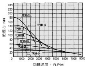
把握力性能曲線 TF3B
